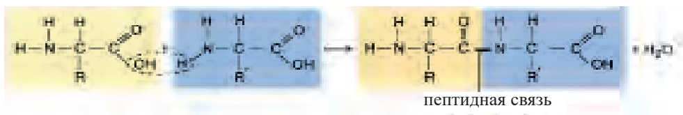
Рис.8. Взаимодействие аминокислот
