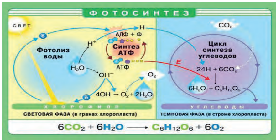
Рис.23. Процесс фотосинтеза.
