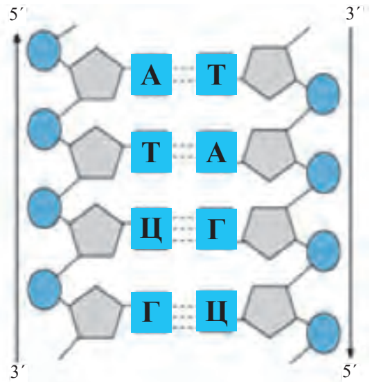
Рис.16. ДНК.
