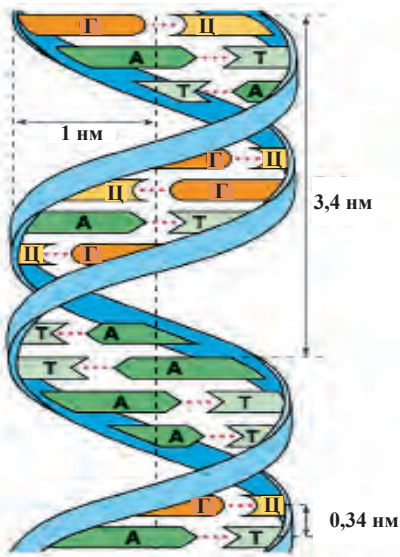
Рис.15. Структура ДНК
