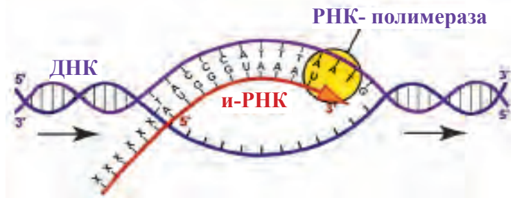
Рис.26. Транскрипция.
