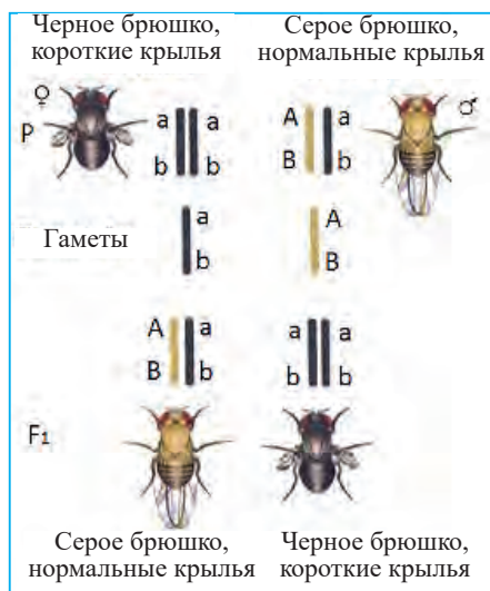
Рис.46. Полное скрещивание.
