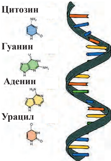
Рис.17. Структура РНК.
